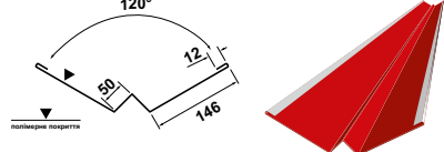
Кошикова ринва трикутна, P=416
