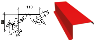
Вітрівниця верхня, P=250
