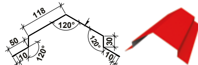
Коньок трапецієвидний, P=416
