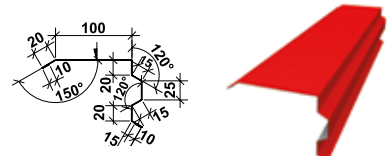
Вітрівниця верхня фігурна, P=250
