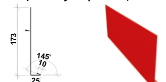
Вітрівниця бічна універсальна, P=208
