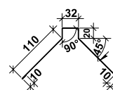
Коньок прямий, P=312
